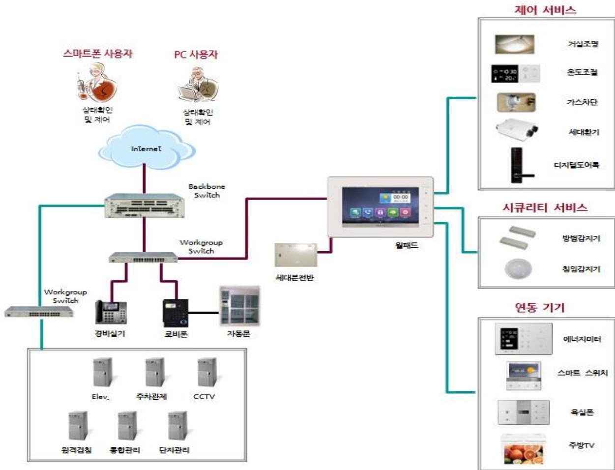
그림 21. 차기 홈네트워크 구성도
